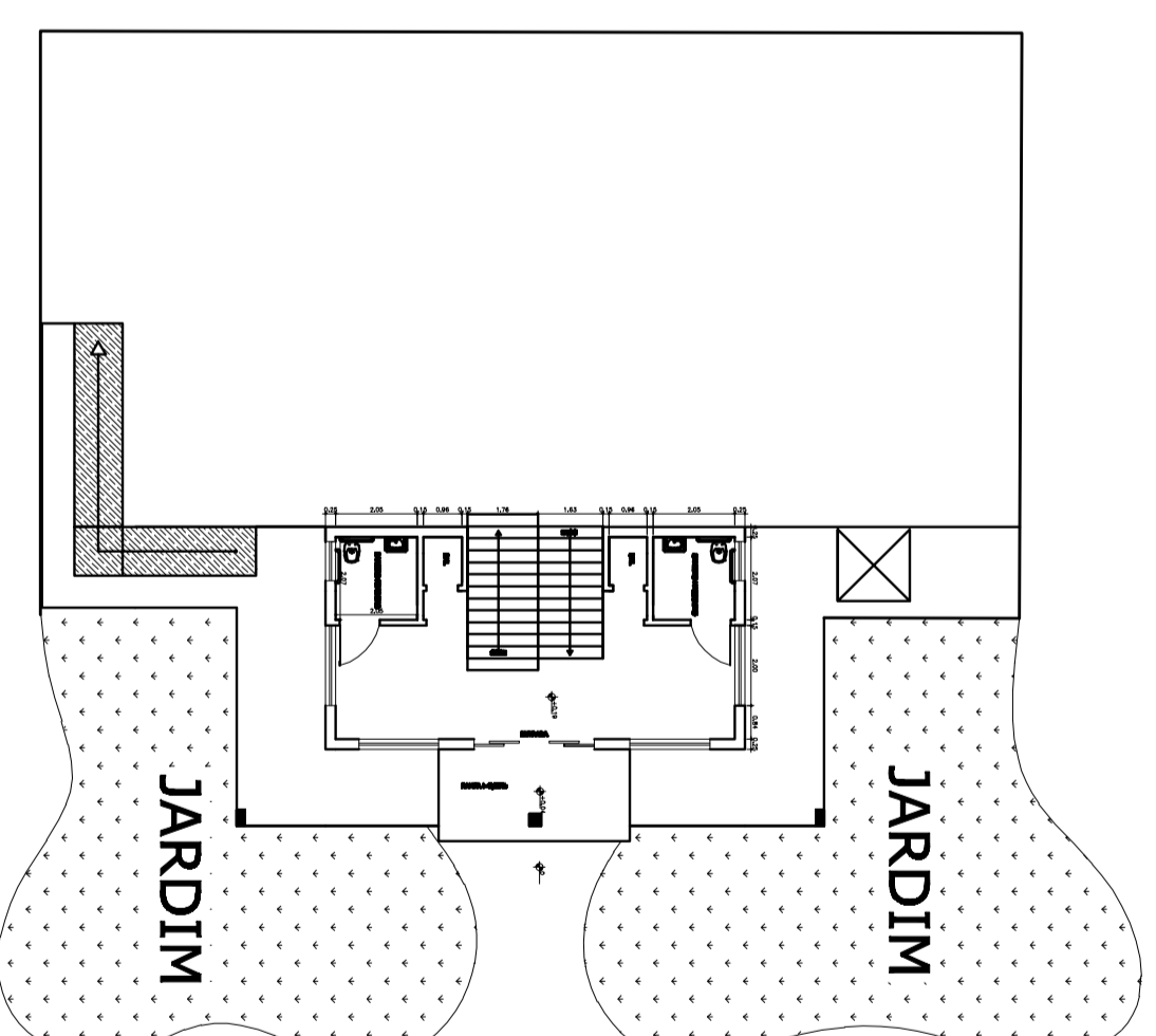
PLANTA DE ADAPTAÇÃO ESCALA 1/200
